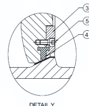
DETAIL Y
